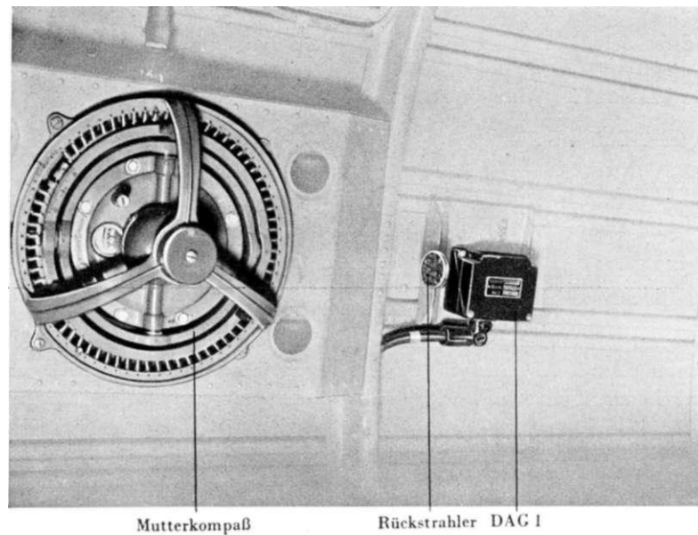
Abb. 19: Dipolanpassungsgerät DAG 1
