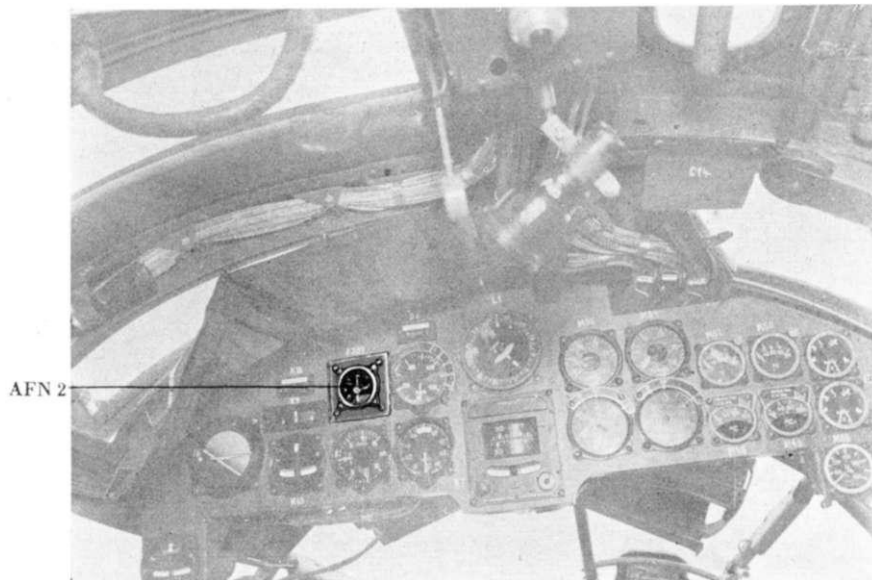
Abb. 6: Anzeigegerät AFN 2
