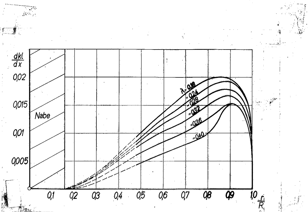
Bild 12. Drehmomentverteilung über dem Schraubenradius bei verschiedenen Fortschrittsgraden ( \beta_d = 25,6^\circ ).
