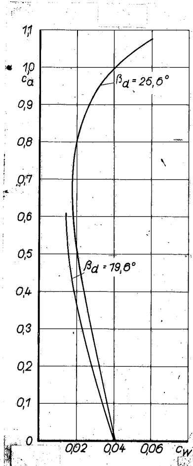
Bild 32. Polaren des Profilschnittes x = 0,7 für zwei Steigungswinkel; Ma < 0,5 .
